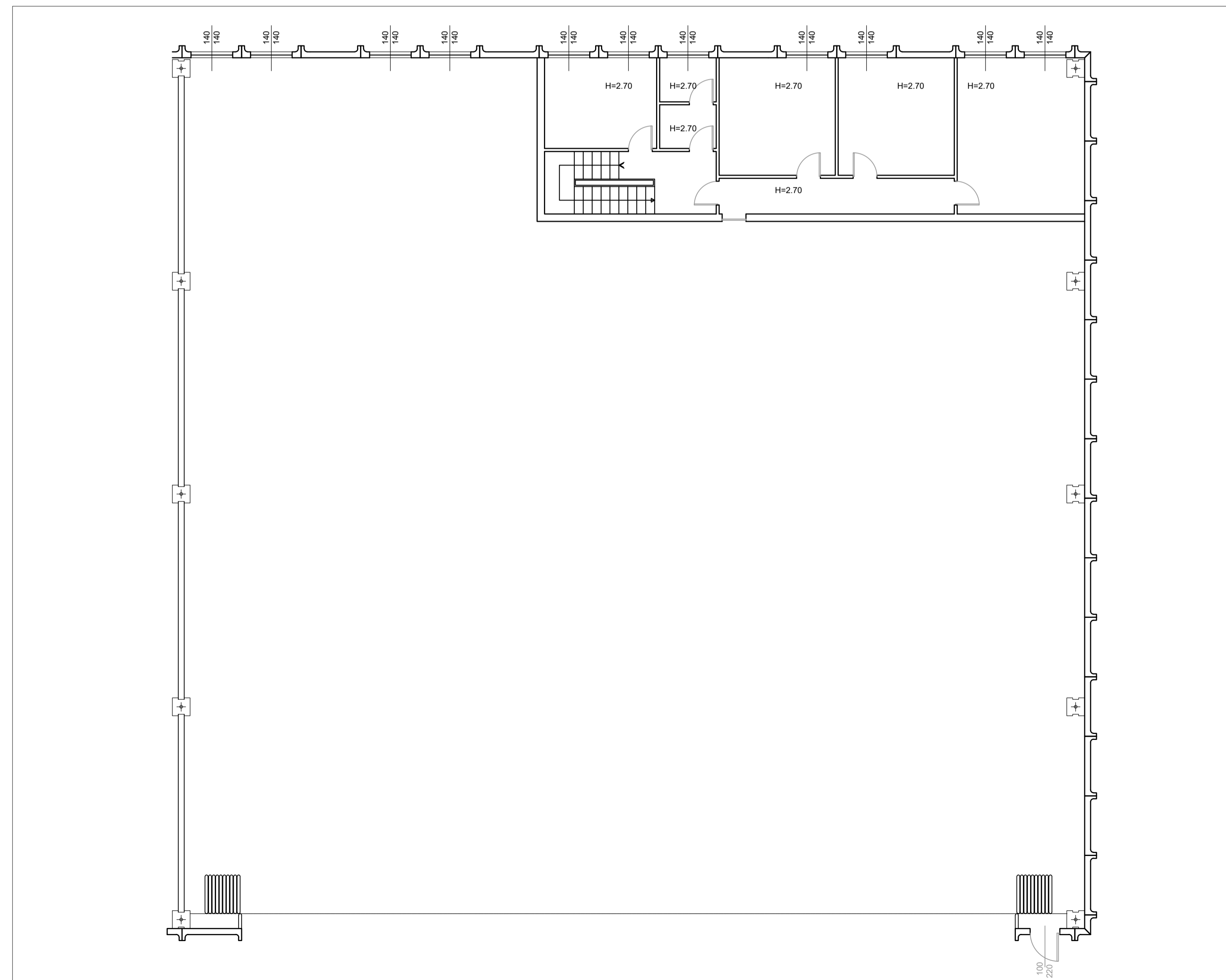
HANGAR - PIANO PRIMO, scala 1:100
